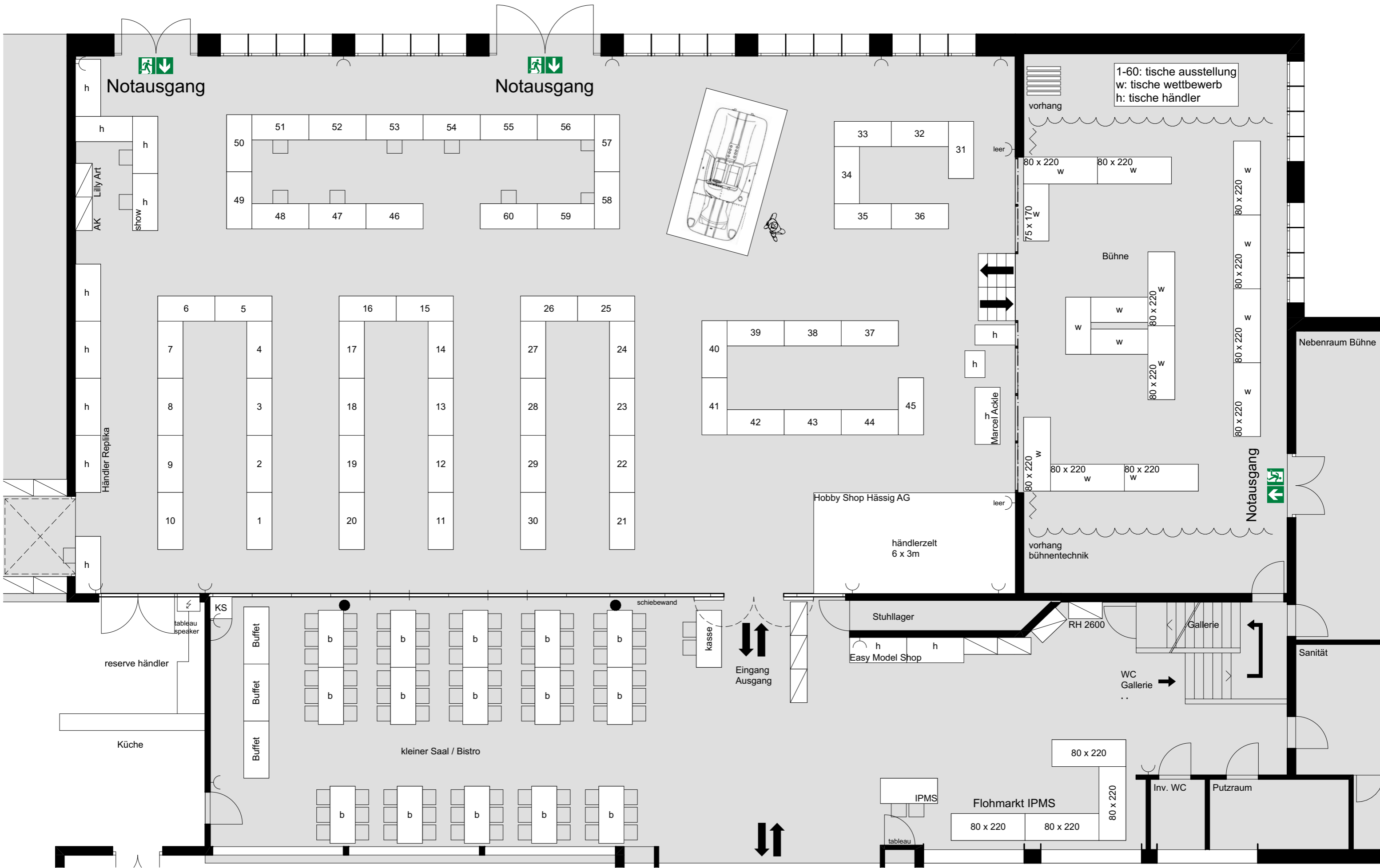
variante 2, ipms sg ausstellung + nationaler wettbewerb 1:100/A3
